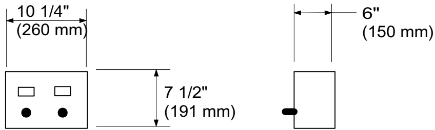
INDICATOR BOX
